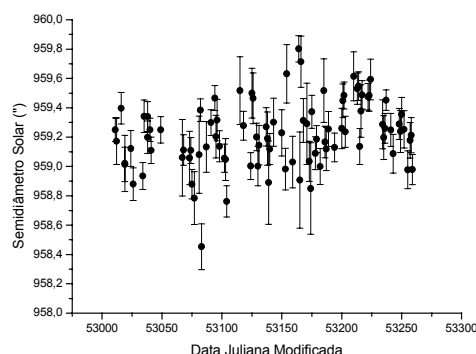
Figura 3. Médias diárias do semidiâmetro solar.
